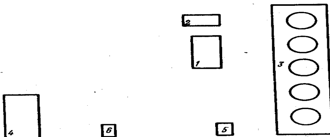
Рис. 4. Типовая схема рабочего места для заполнения штангласов лекарственными средствами
